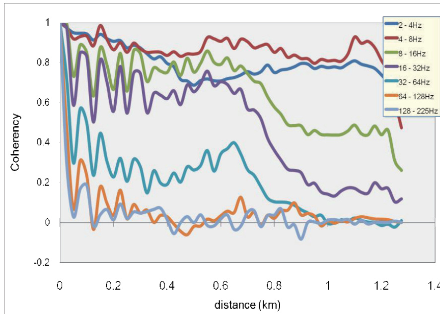
図9. 周波数ごとの直達P波の観測点波形相関（上下動成分）。横軸は観測点間距離。すべての組み合わせを取り、距離ごとに平均して求めた。
