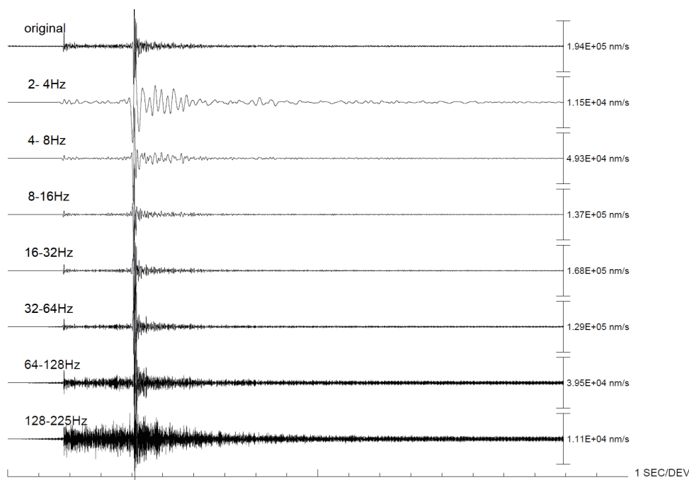
図8. 図7で示した波形のバンドパスフィルター処理波形.
