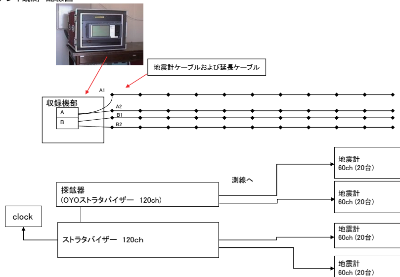
図2. 観測システムのダイアグラム. 測線は60 ch CDPケーブル4本で構成され, 240 ch (80点3成分)を探鉱器で収録した. イベント収録はトリガー信号を同期することで同時トリガを行った. トリガは測線上の6点におけるSTA/LTAのANDによって判定した. サンプル間隔は時期により1,2,4 msecと変えて収録した. データ長はこれらのサンプル間隔によって変わり, 16, 32, 64秒である.
