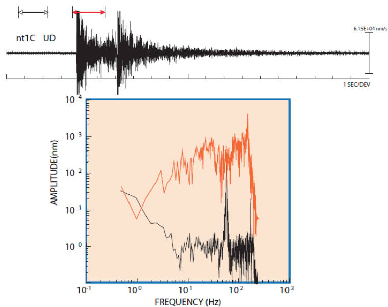
図7. アレイの1点における上下動地震計記録（上図）とノイズ部分（黒線）と直達P波部分（赤線）の振幅スペクトル（下図）。上図中での矢印はスペクトルウィンドウを示す。
