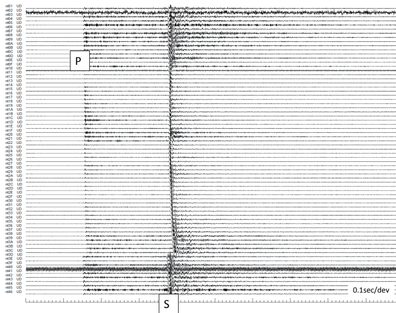
図6. 観測波形例。上下動地震計の波形を示す。図中のP, Sは直達P波, S波の部分を示す。
